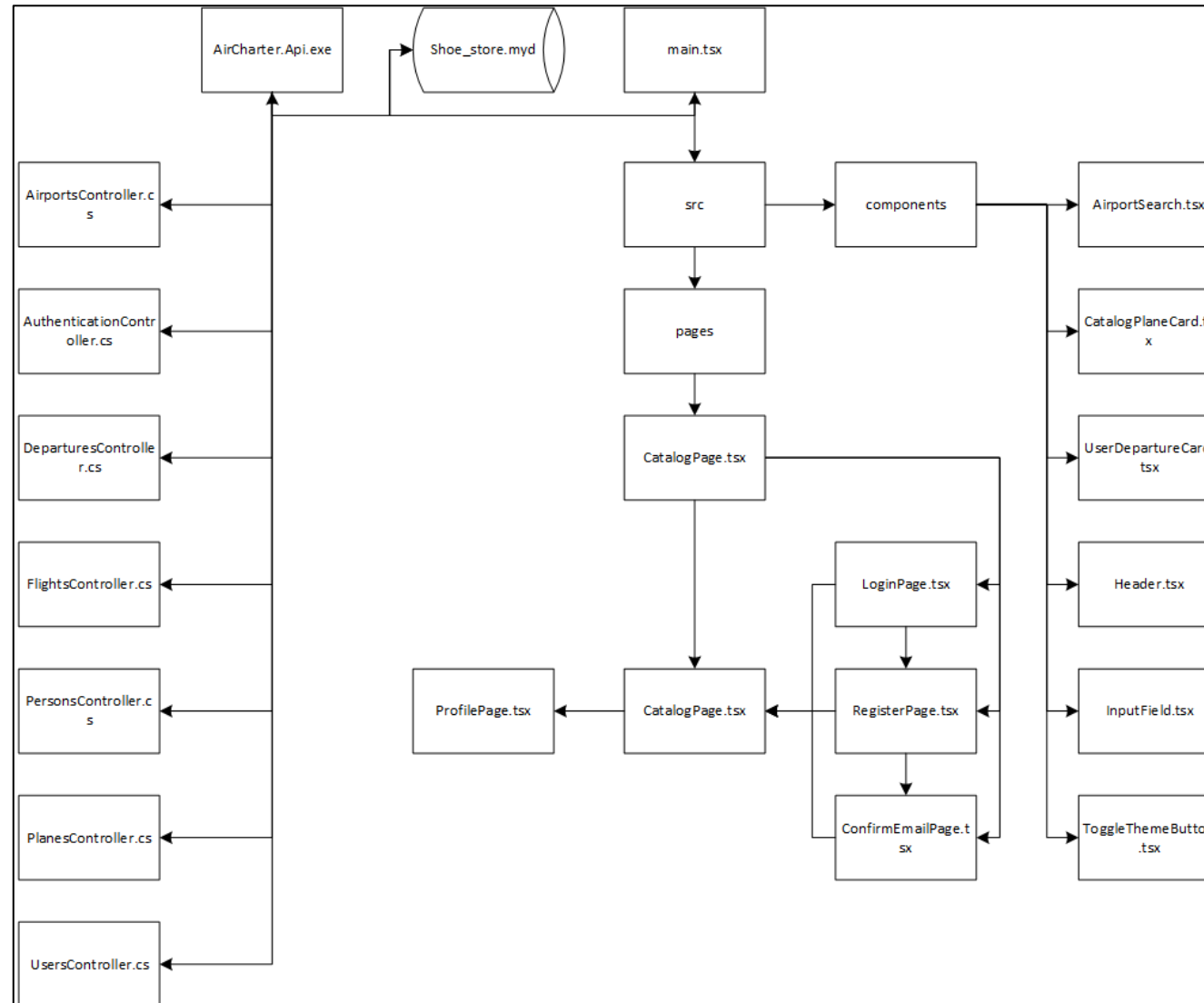
Рисунок Г.1 – Модульная схема приложения
