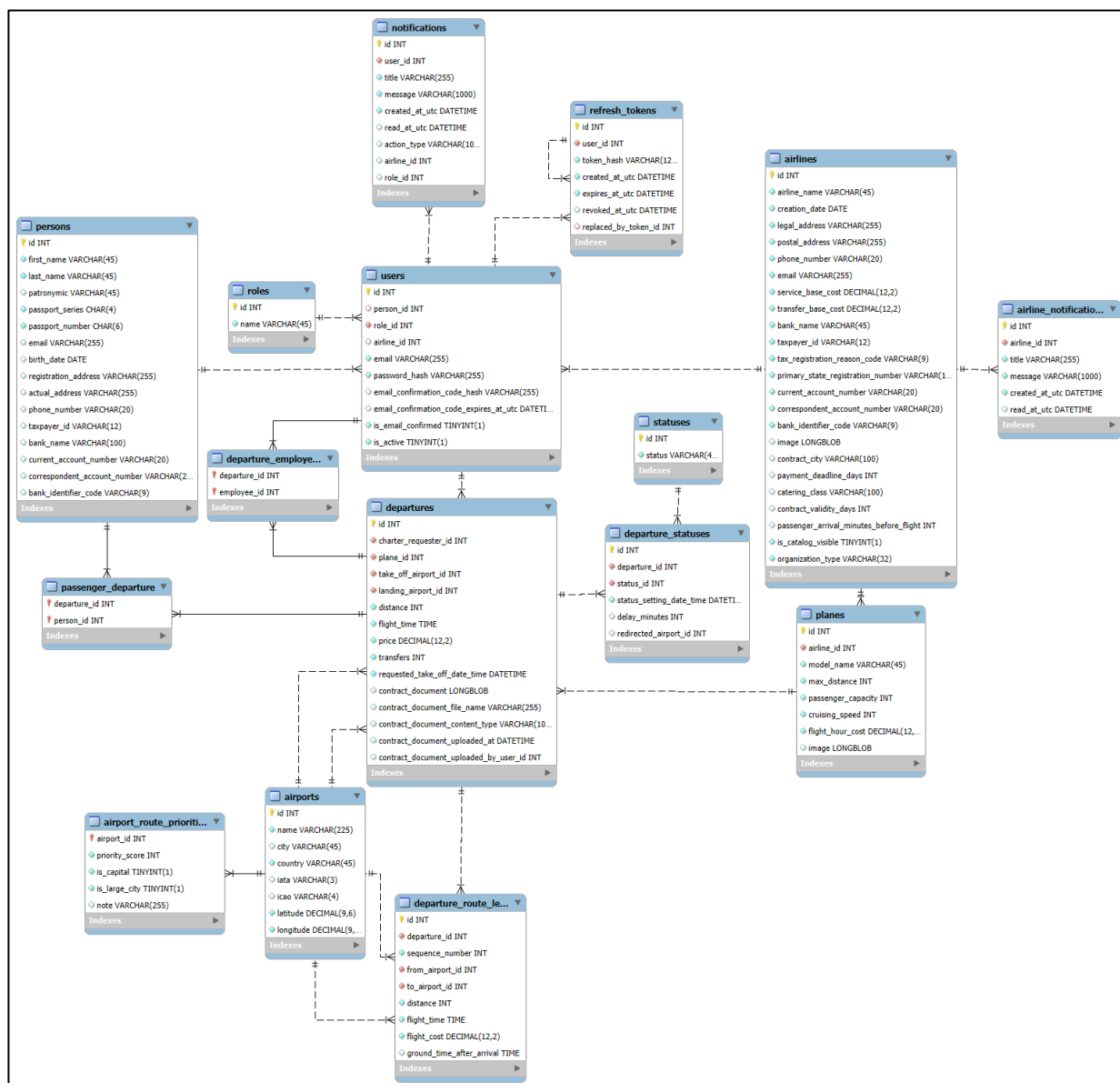
Рисунок 1.6.1 – ER диаграмма БД
