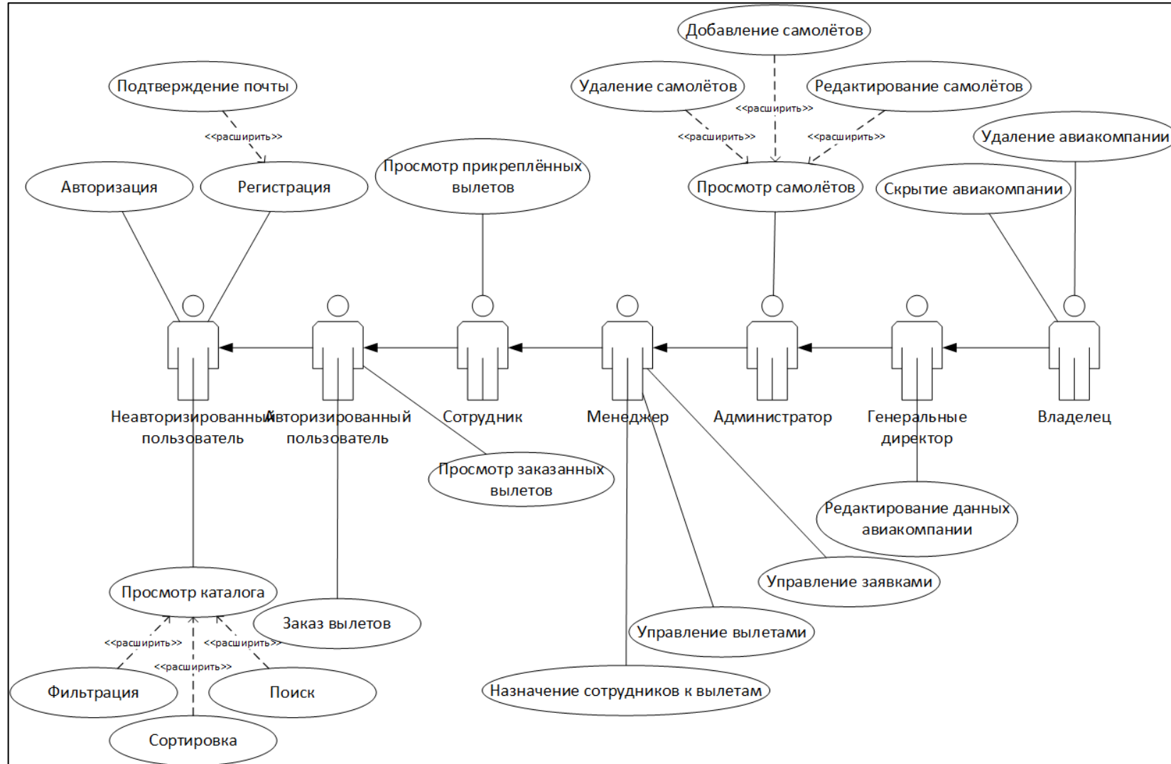
Рисунок А.1 – Диаграмма вариантов использования
